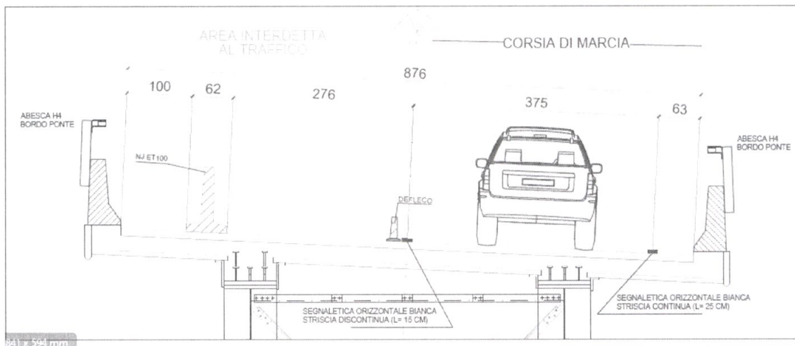
Interventi su carreggiata nord - cantiere su una corsia
